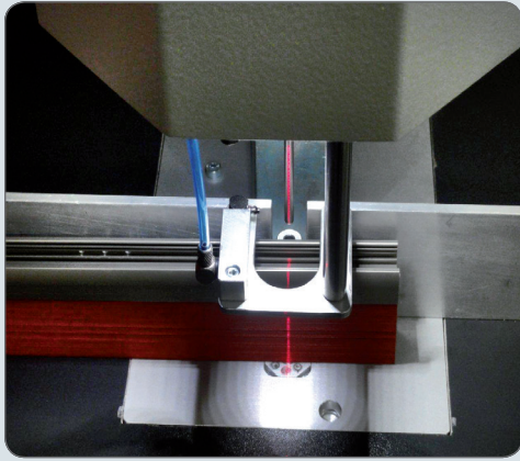
Strichlaser für Stoffpaket-Positionierung Line laser for positioning fabric stack.
